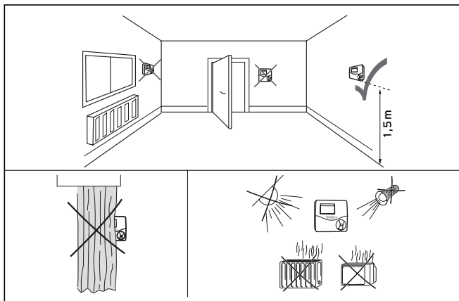
Afb. 8.1 Montageplaats kiezen
