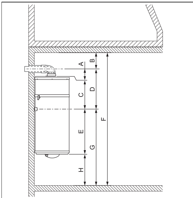
Afmetingen van een gedeeltelijk leidingsysteem zonder driepotige standaard
