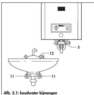
Afb. 5.1: koudwater bijmengen
