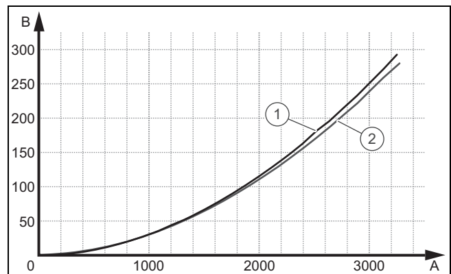
A Volumenstrom (l/h) 1 Warmerwasserkreis B Druckverlust (mbar) 2 Heizkreis
