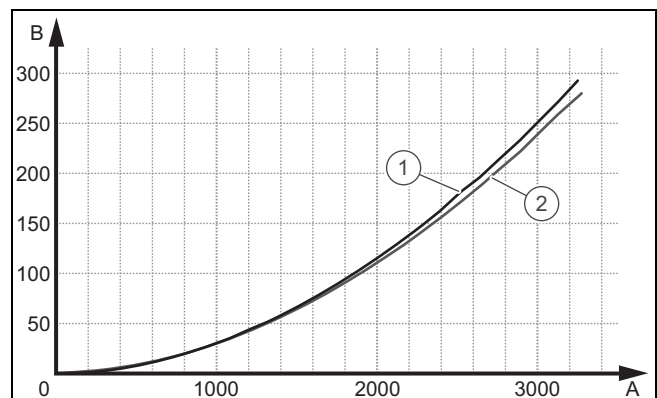
A Débit volumique [l/h] 1 Circuit sanitaire B Pertes de charge [mbar] 2 Circuit chauffage
