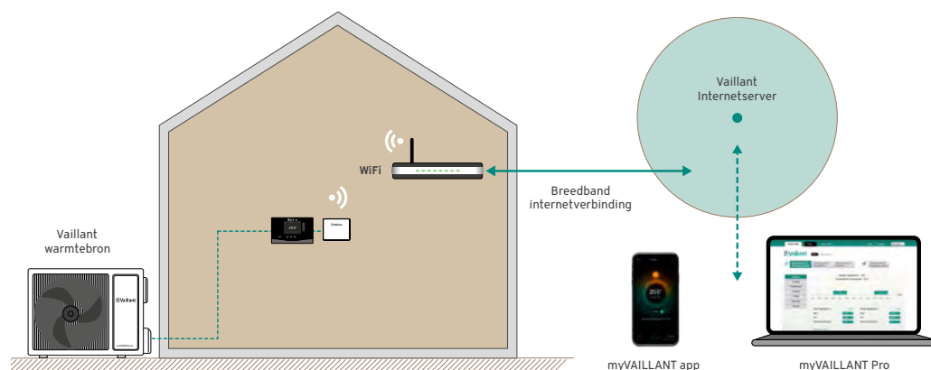
In bovenstaande afbeelding ziet u hoe de myVAILLANT connect VR 940f service werkt en dat de gateway gebruik maakt van de zwaar beveiligde Vaillant internetserver.
